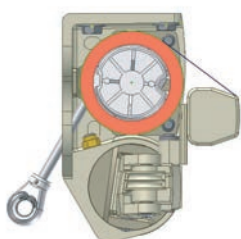
Pose plafond avec sortie treuil à l'arrière du store
